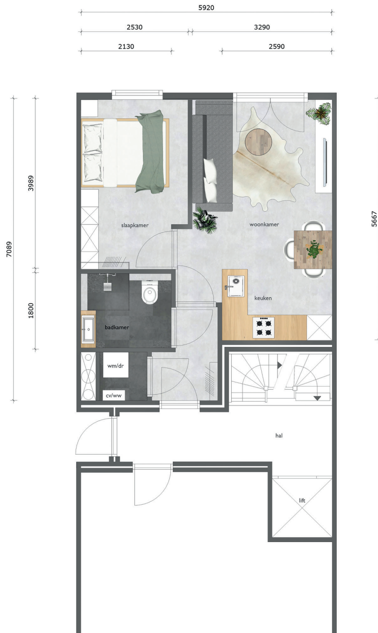
SITUATIE
